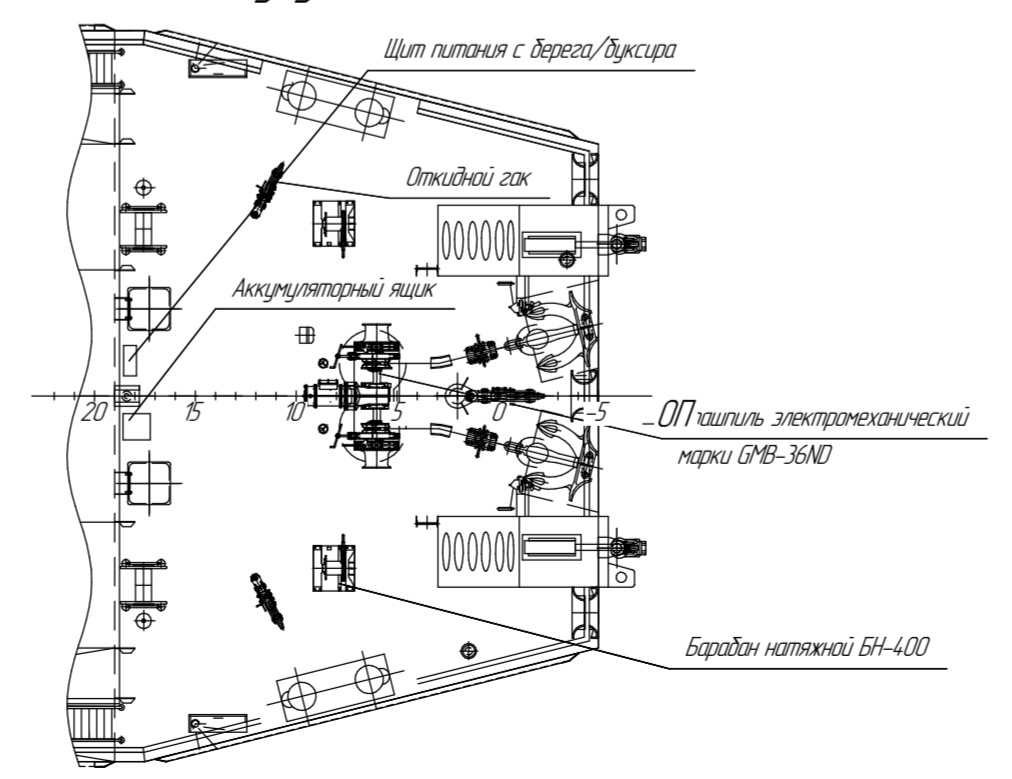
Вид на палубу бака без навеса
