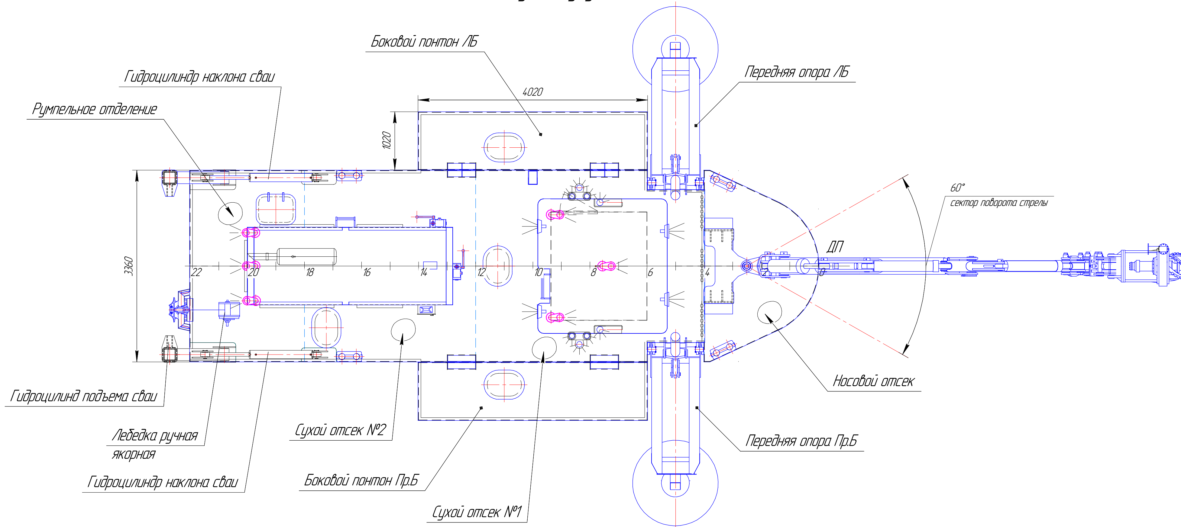
Вид на главную палубу
